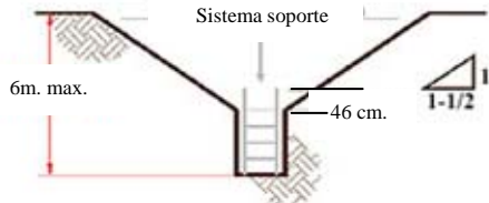
PORCION MAS BAJA VERTICALMENTE CON TALUD CON SOPORTE TIPO DE SUELO C
