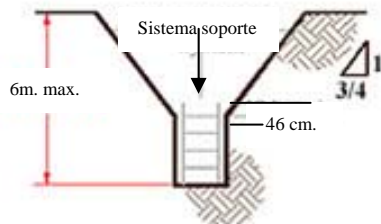
PORCION MAS BAJA VERTICALMENTE CON TALUD CON SOPORTE
